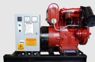
CAE 12,5/11 BASE BOUNOUS Grupo electrógeno monofásico diésel. 12,5 KVA potencia Stand By, 11 KVA potencia PRIME.
