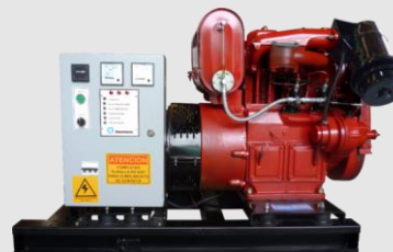
CATE 15/13,5 BASE BOUNOUS Grupo electrógeno trifásico diésel. 15 KVA potencia Stand By, 13,5 KVA potencia PRIME.
